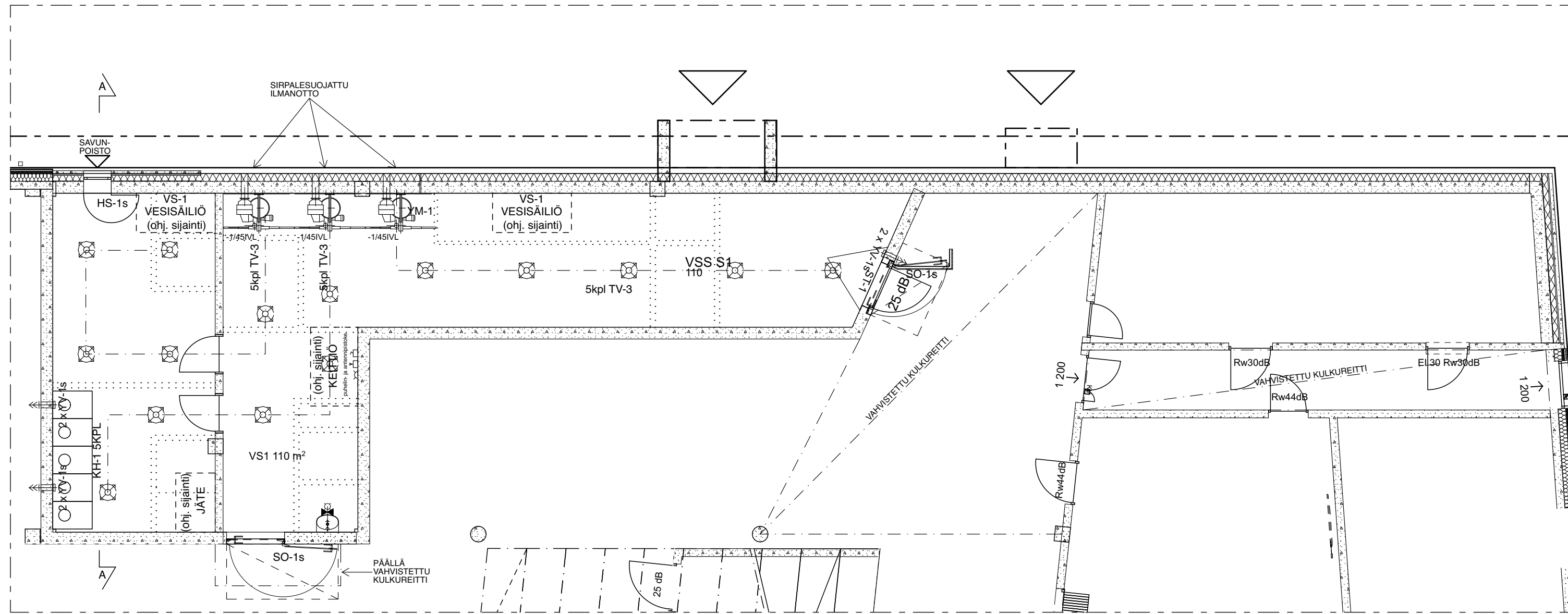
POHJA 1:100
