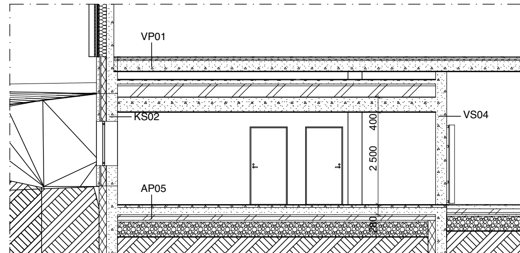
LEIKKAUS A-A 1:100
